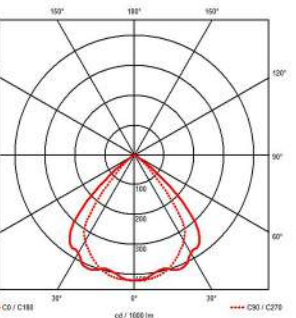
Atlas 1 Louver 2x39W
