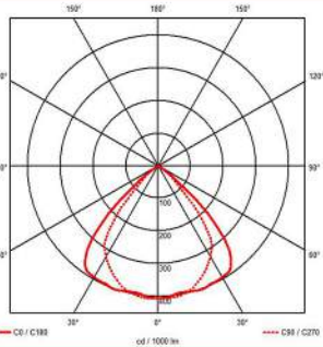
Atlas 1 Louver 2x21W
