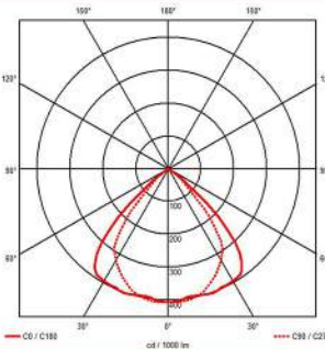
Atlas 1 Louver 2x24W
