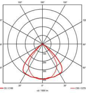
Atlas 1 Louver 1x39W
