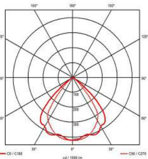
Atlas 1 Louver 2x35W
