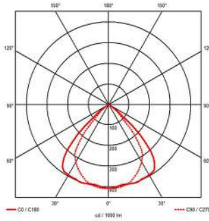
Atlas 1 Louver 1x35W
