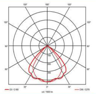
Atlas 1 Louver 2x80W
