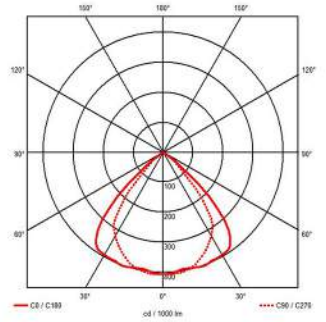
Atlas 1 Louver 1x80W
